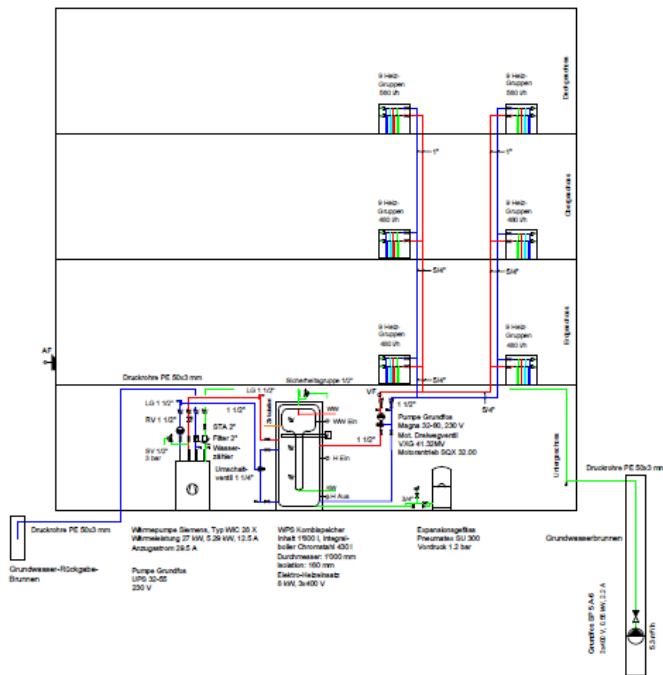
Schema Heizung
