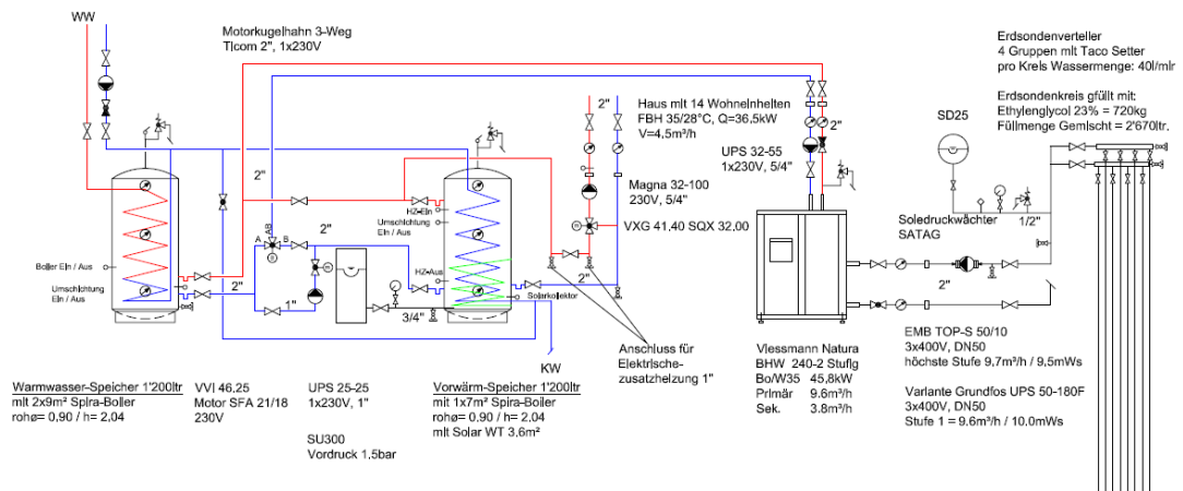
Schema Heizung
